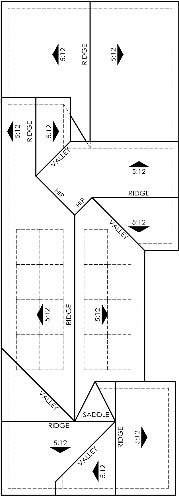
ROOF PLAN 4B OVERHANG : 12" RAKE : 12" ROOF PITCH : 5:12 U.N.O
