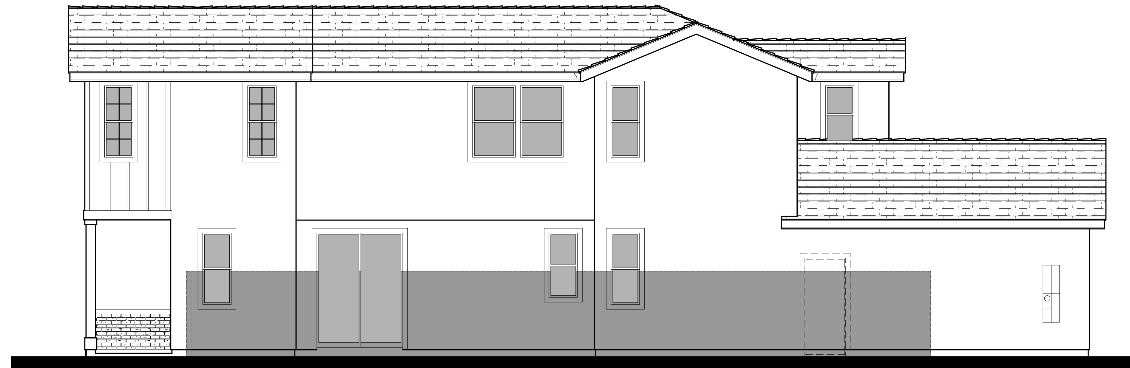
Right Elevation
