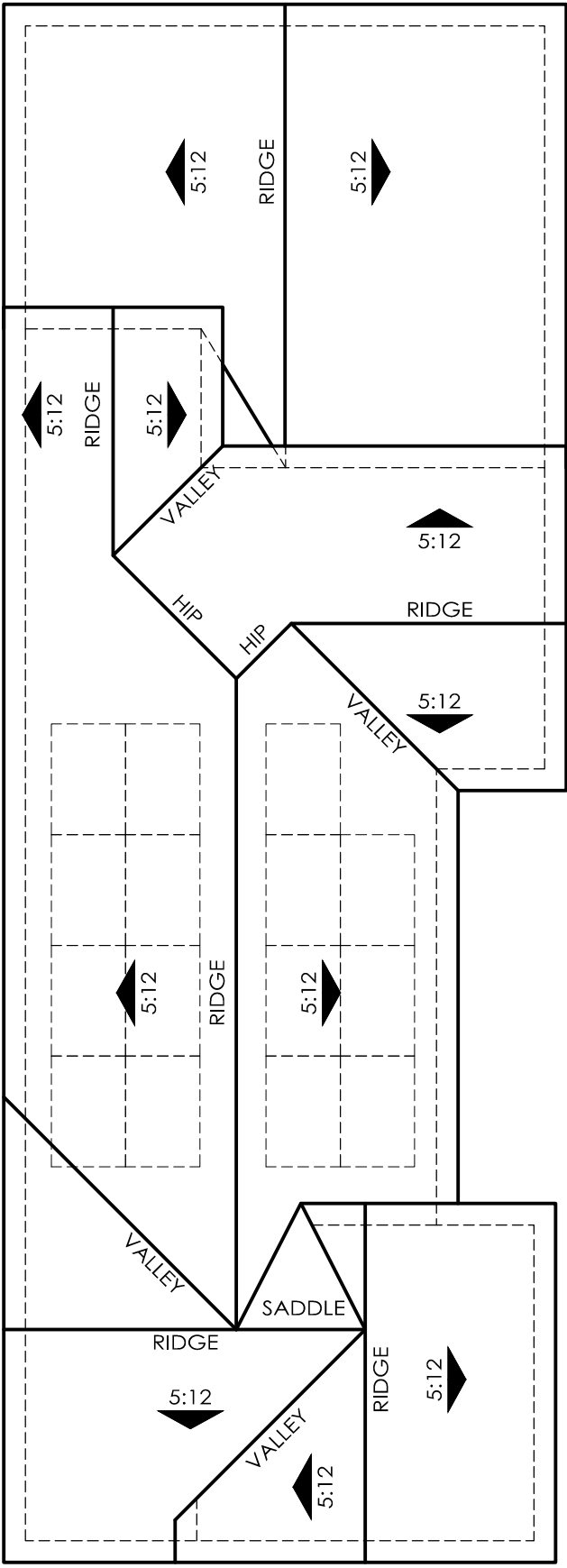
ROOF PLAN 4C OVERHANG : 12" RAKE : 12" ROOF PITCH : 5:12 U.N.O 0 4 8 16
