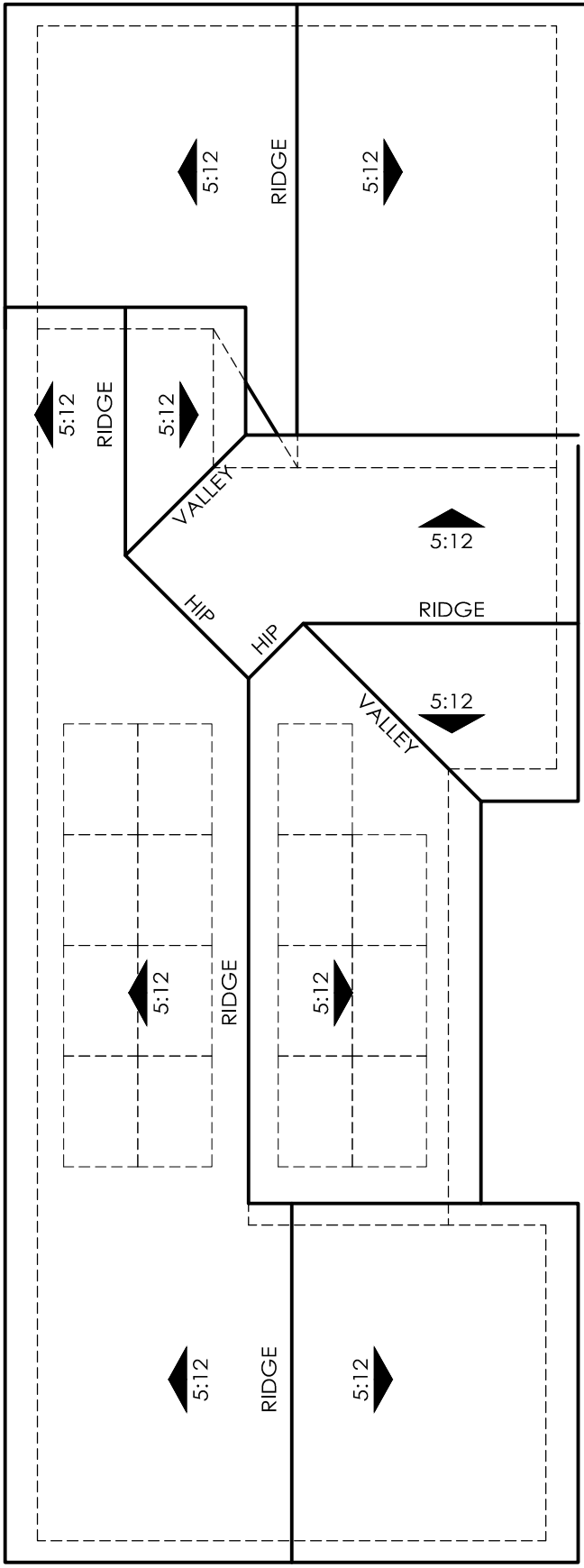
ROOF PLAN 4A OVERHANG : 18" RAKE : 12" ROOF PITCH : 5:12 U.N.O 0 4 8 16
