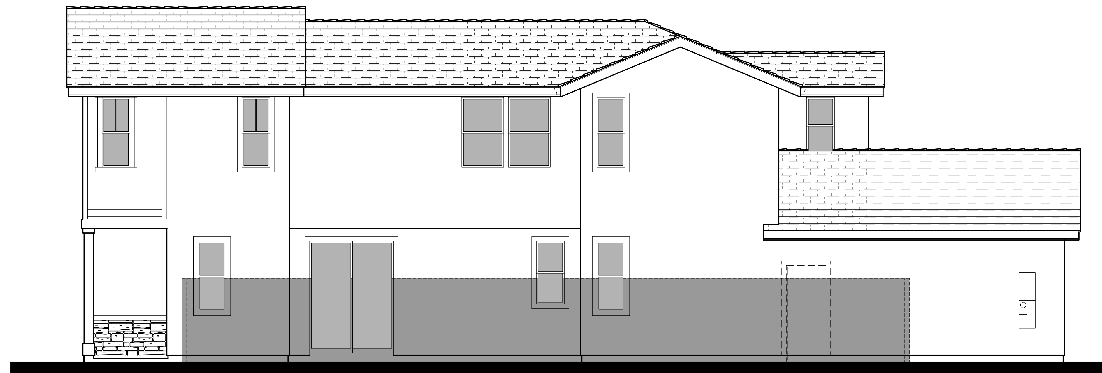
Right Elevation
